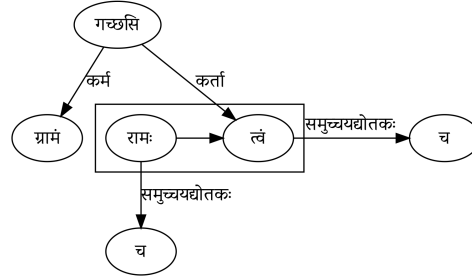
चित्रम् 4.11: रामः च त्वं च ग्रामं गच्छसि।
