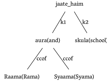
चित्रम् 4.9: Hindi Treebank
