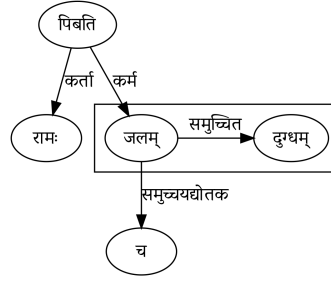
चित्रम् 4.14: रामः दुग्धं जलं च पिबति।
