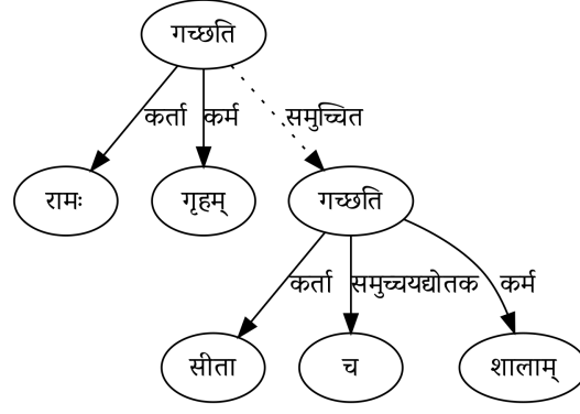
चित्रम् 4.17: रामः गृहं गच्छति सीता च शालाम्।
