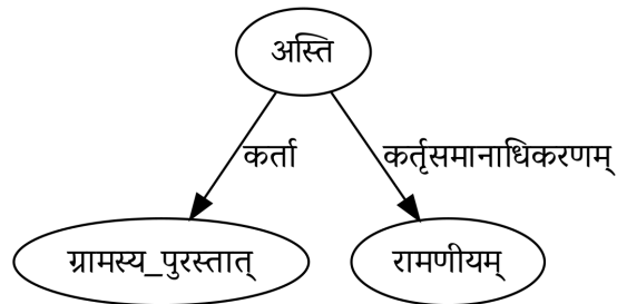
चित्रम् 3.10: ग्रामस्य पुरस्तात् रमणीयम् अस्ति
