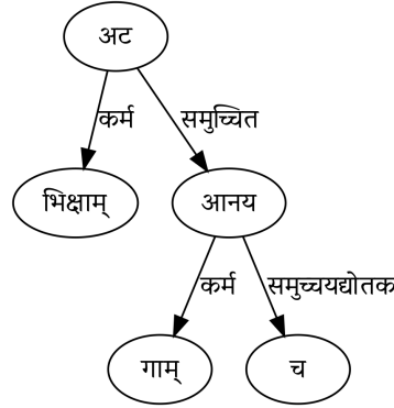
चित्रम् 4.16: भिक्षाम् अट गां च आनय।
