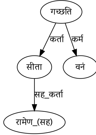
चित्रम् 3.7: सहार्थसम्बन्धस्य आर्थिकस्तरे विश्लेषणम्
