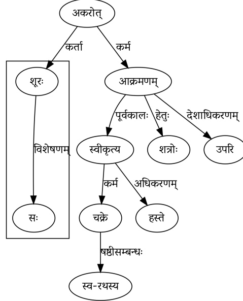
चित्रम् 7.9: सः शूरः स्व-रथस्य चक्रे हस्ते स्वीकृत्य शत्रोः उपरि आक्रमणम् अकरोत्।
