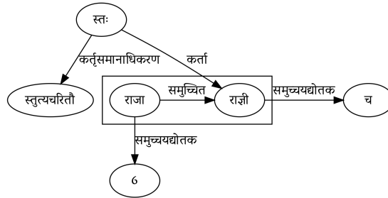
चित्रम् 4.15: राजा राज्ञी च स्तुत्यचरितौ स्तः।
