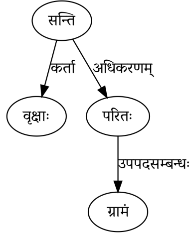
चित्रम् 3.2: विभक्त्याधारेणोपपदवर्गीकरणे विश्लेषणम्
