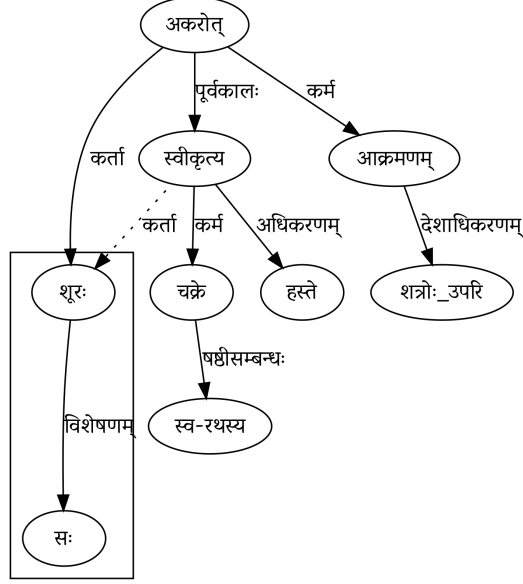
चित्रम् 7.11: सः शूरः स्व-रथस्य चक्रे हस्ते स्वीकृत्य शत्रोः उपरि आक्रमणम् अकरोत्।
